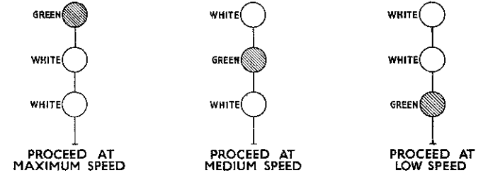
Fig. 3 Proceed indications
